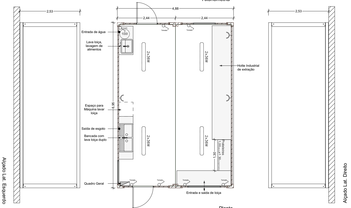
Planta
